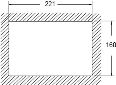
开孔尺寸
